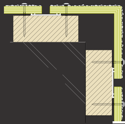
Hoekoplossing met Colorstone® Textures hoekstuk
