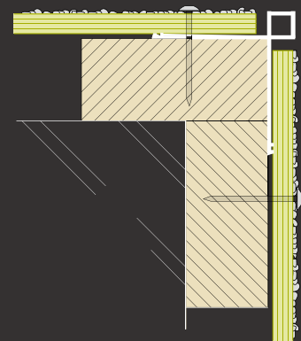
Hoekoplossing met kunststof profiel
